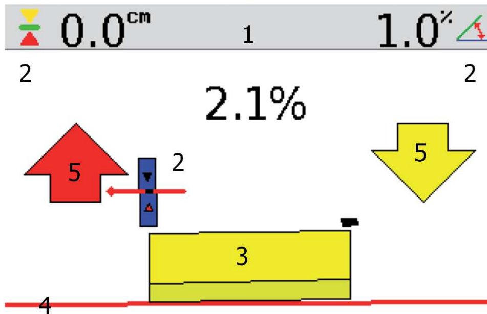
Figuur 2: Laser en cross slope sensor geselecteerd
